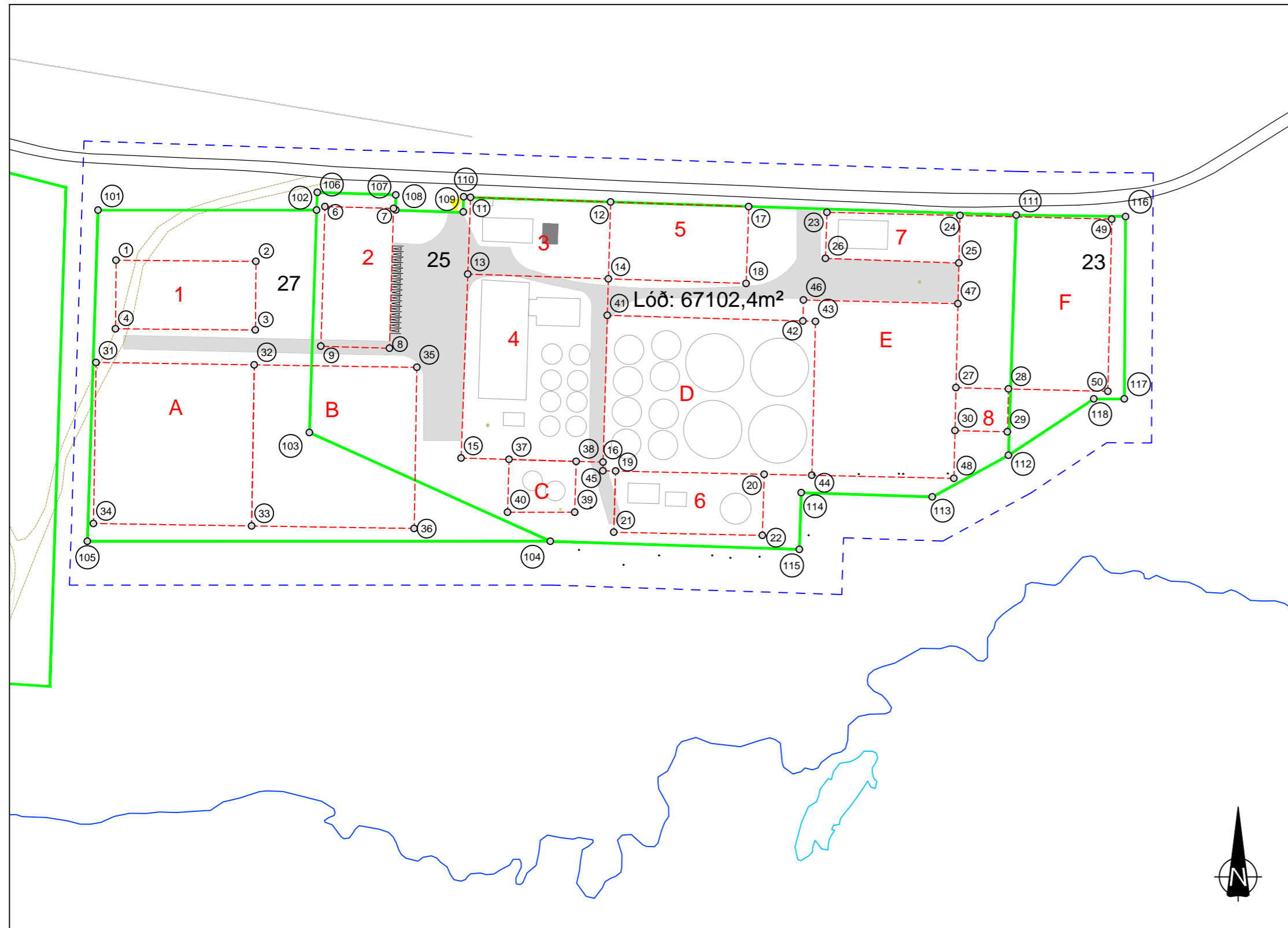
Deiliskipulagsuppráttur 1:2000
